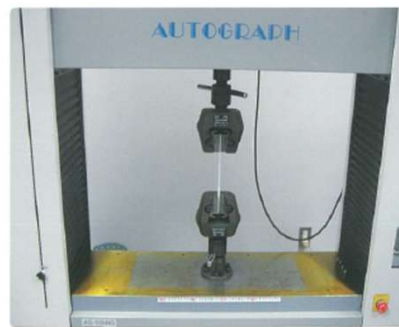
JIS K 7164 引張り試験
